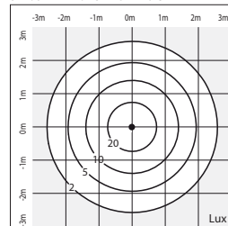
S7168 - 1x 26 FSM GX24 d-3 H=1 m
