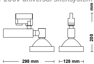
Spotlight för 230V universal skensystem av Global typ.
